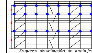
Esquema distribución de anclajes
